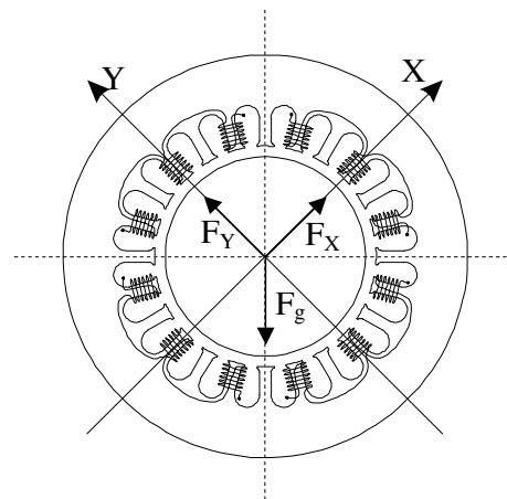
Fig. 8. Configuration of the rotor in the AMB system.
