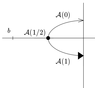
Fig. 2. Points singuliers de g
